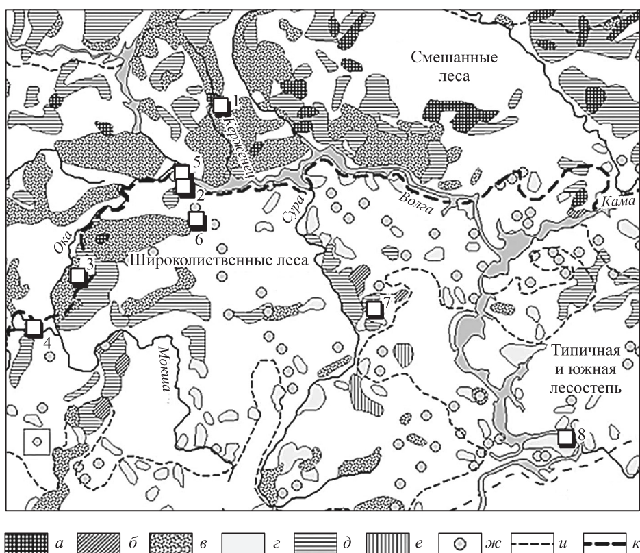
Рис. 1. Растительный покров Среднего Поволжья (по: Растительность..., 1987) и схема расположения экспериментальных полигонов.
