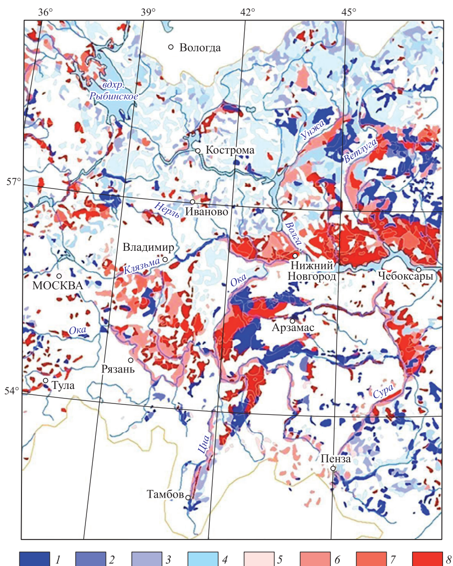
Рис. 3. Удельный баланс углерода в растительных формациях Волжского бассейна на 2200 г. по прогнозно-климатической модели E GISS (умеренный термоаридный тренд). Масштаб 1 : 4 200 000. Карта рассчитана и составлена Л. С. Шарой. Ареалы даны по картам лесов (Карта..., 1974; Растительность..., 1987).
